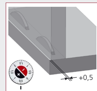
Rücksprung eines Werkstückes
