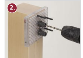
2. Kontur übertragen, Schablone ausrichten und bohren
