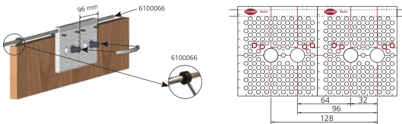
Möbelgriff-Löcher und Reihenlochbohrungen im 32 mm Raster
