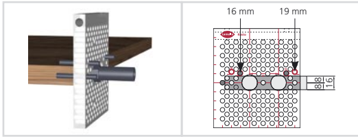
Mittiges Bohren in 16 und 19 mm Platten
